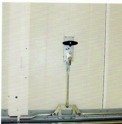
Vergrendeling kanteldeurblad
