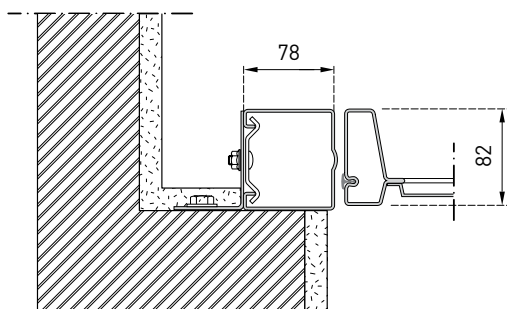
blokkozijn
