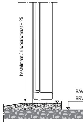
Detail A: zonder aanslag
